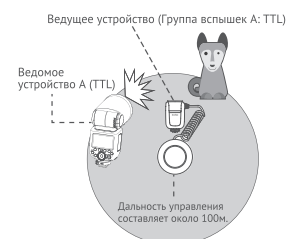
Съемка в режиме автовспышки с одним ведомым устройством
