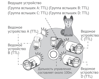
Съемка в режиме автовспышки с четырьмя ведомыми устройствами
