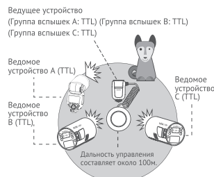
Съемка в режиме автовспышки с тремя ведомыми устройствами
